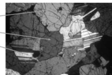
Gabbro de la croûte océanique Banque Nationale de photos en SVT - Lyon www2.ac-lyon.fr/enseigne/biologie/photosql/photos.php
