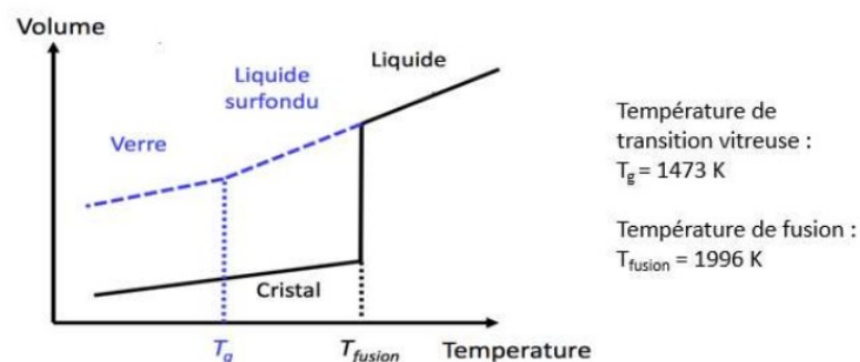
Document 2. Évolution du volume d'un échantillon de silice lors d'un changement d'état.
