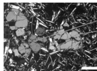
Basalte de dorsale océanique http://www.lppp.fr/jr/Catherine Mével
